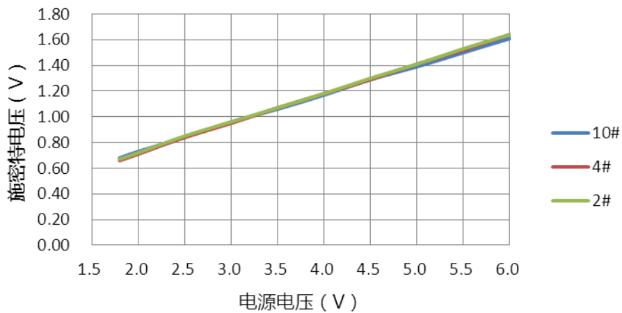
VIH3电压VS电源电压@SMT关闭
