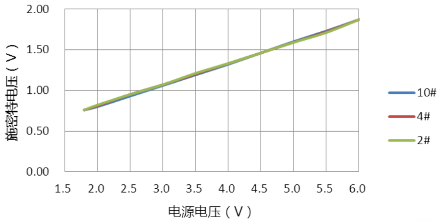
VIH2电压VS电源电压@SMT开启, 阈值选择配置项2
