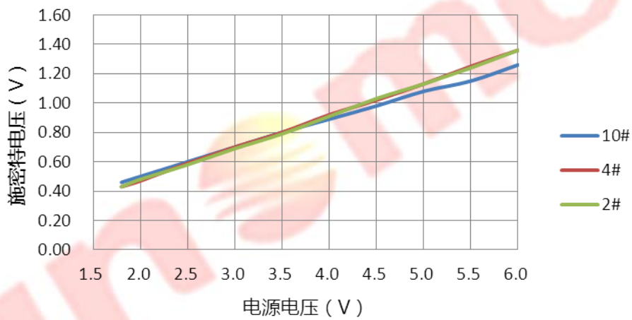
VIL2电压VS电源电压@SMT开启, 阈值选择配置项2
