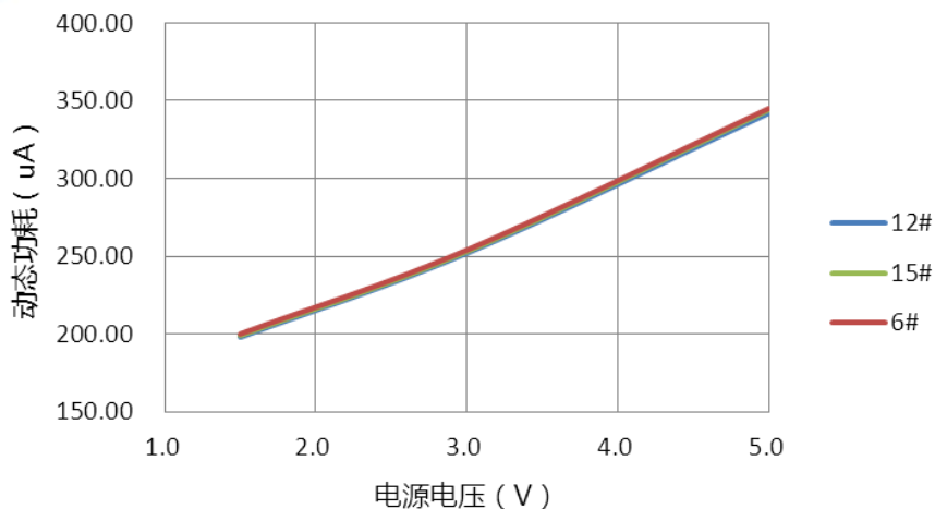
IDD动态功耗VS电源电压@FCPU=227.5K@HIRC=455K
