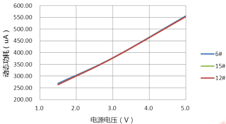
IDD动态功耗VS电源电压@FCPU=1M@HIRC=2M
