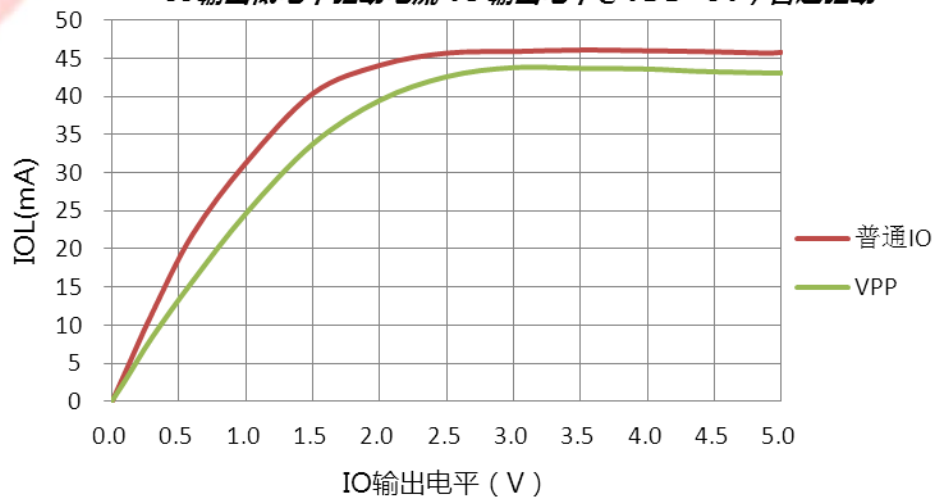
IO输出低电平驱动电流 VS 输出电平@VDD=5V, 普通驱动
