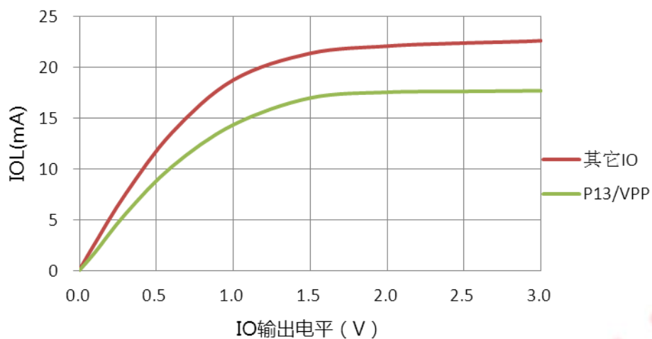
IO输出低电平驱动电流 VS 输出电平@VDD=3V, 普通驱动
