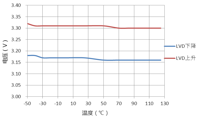
3.2V LVD上升下降电压温度变化曲线
