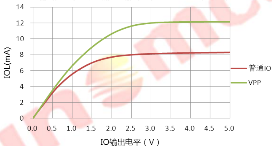
IO输出低电平驱动电流 VS 输出电平@VDD=5V, 弱驱动
