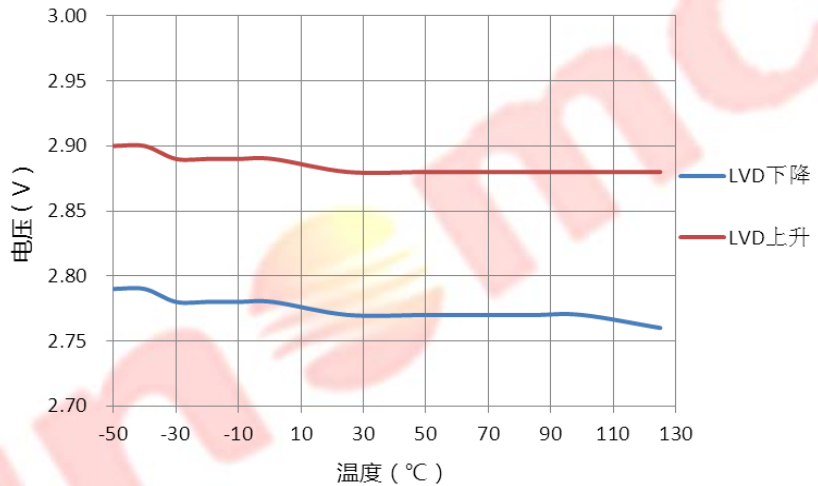
2.8V LVD上升下降电压温度变化曲线
