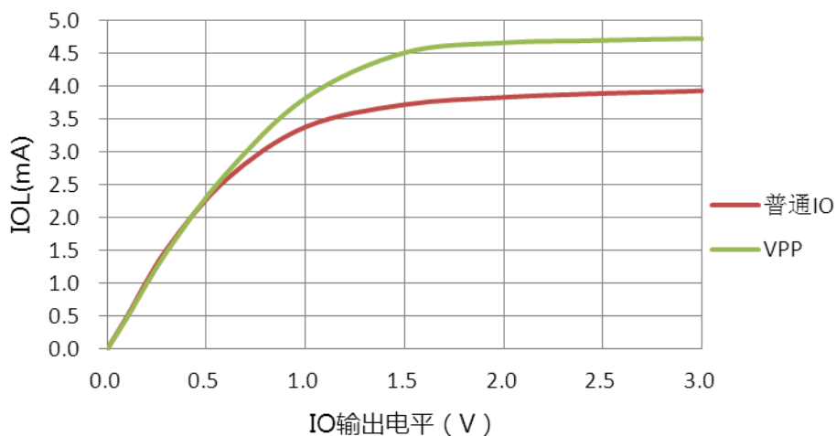
IO输出低电平驱动电流 VS 输出电平@VDD=3V, 弱驱动
