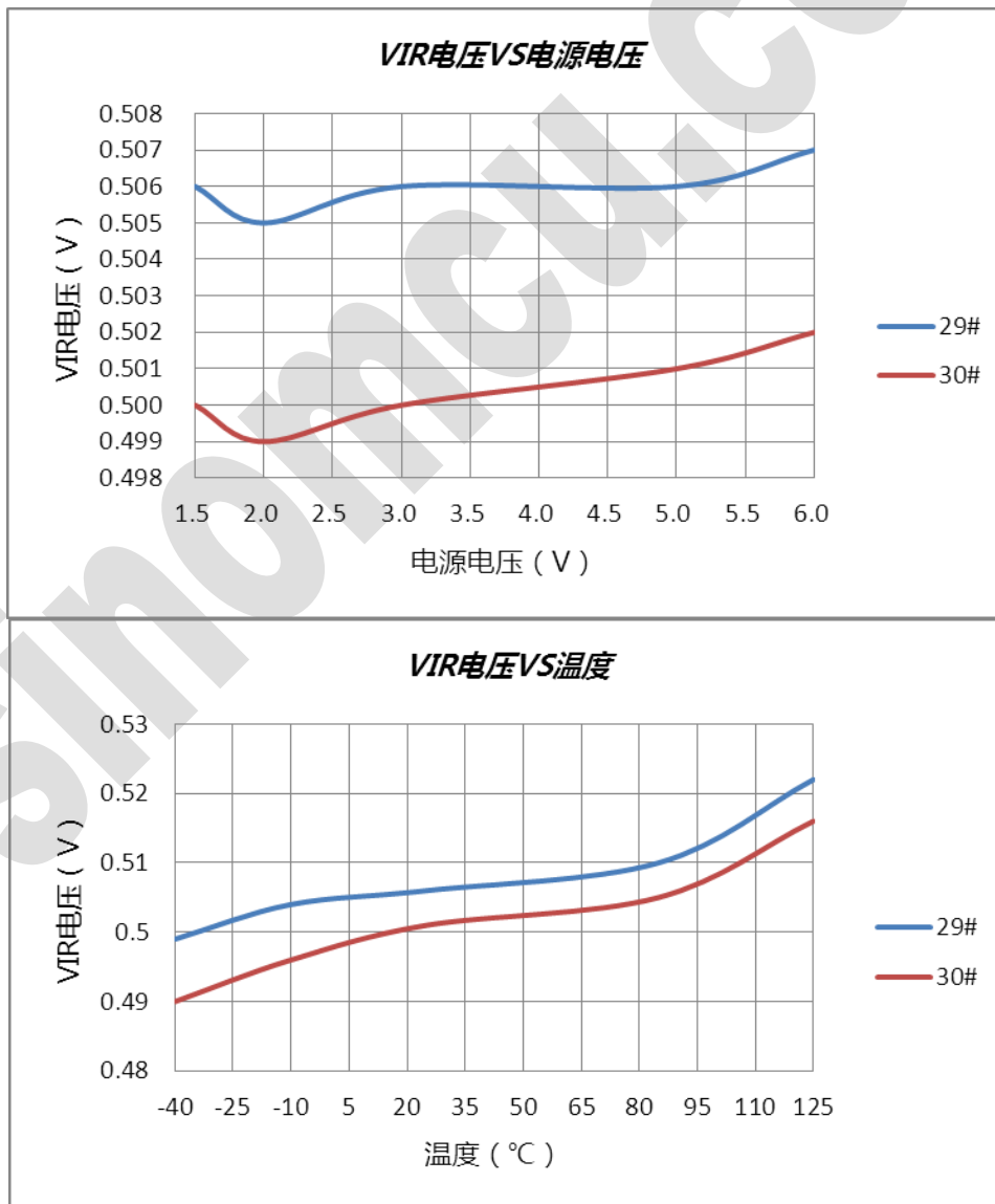
VIR 电压 VS 电源电压/温度
