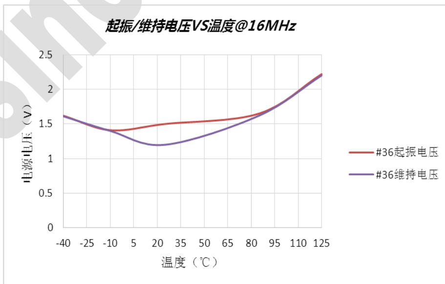
XTAL 起振/维持电压 VS 温度
