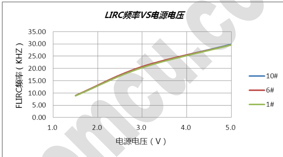
LIRC 频率 VS 电源电压
