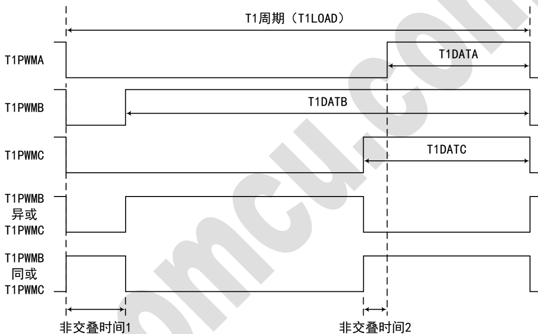
PWM1 互补波形示意
