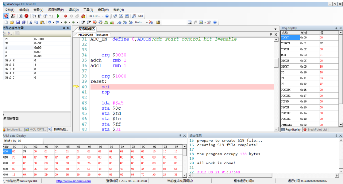
图 26 进入仿真模式
