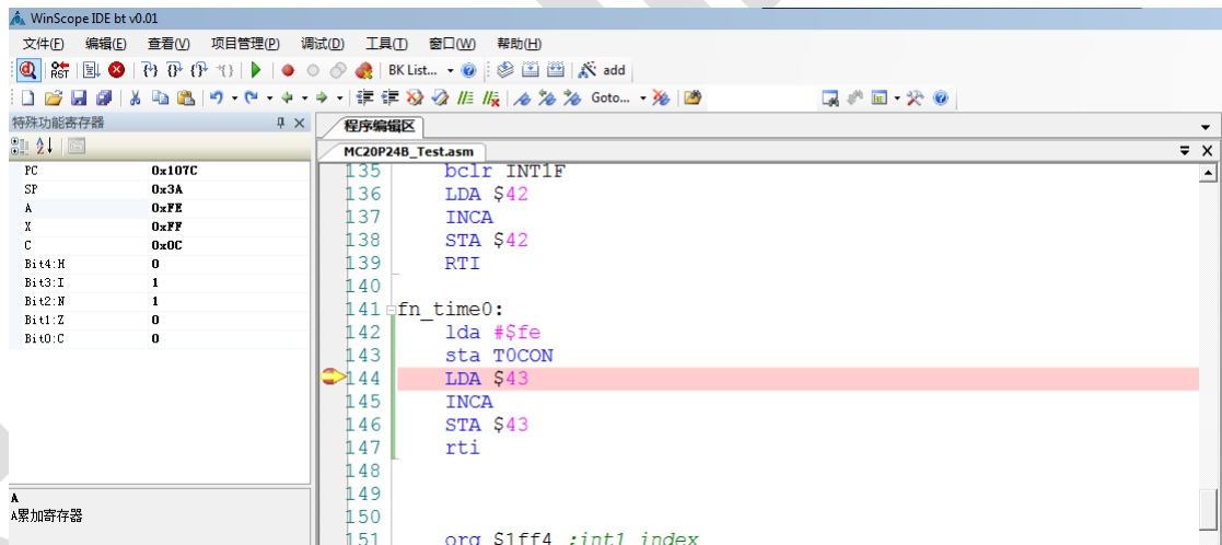
图 27 PC 停留在断点处
