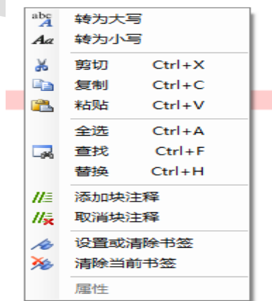
图 2.4 右键菜单
