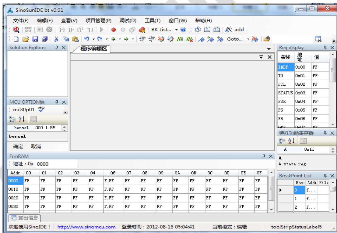
图 19 SinemcuIDE 界面
