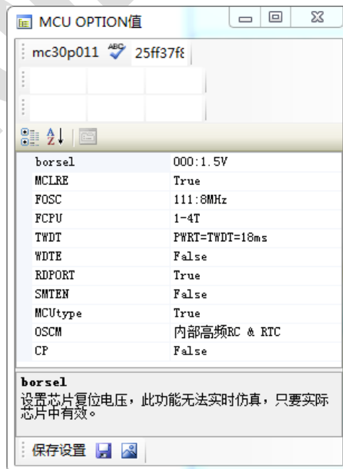
图 37 OPTION 设置
