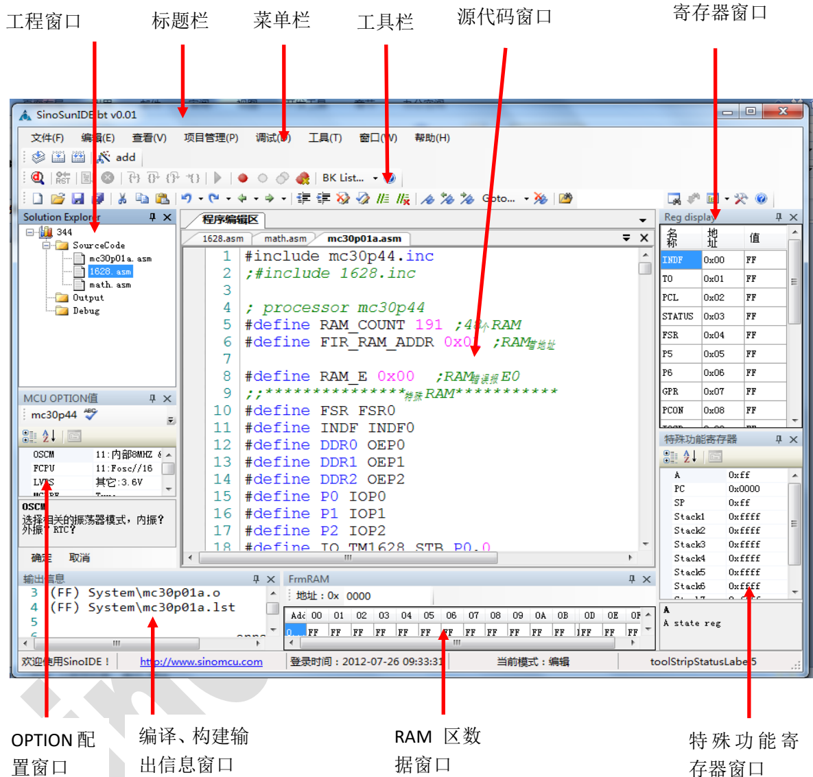
图 2 SinemcuIDE 主界面
