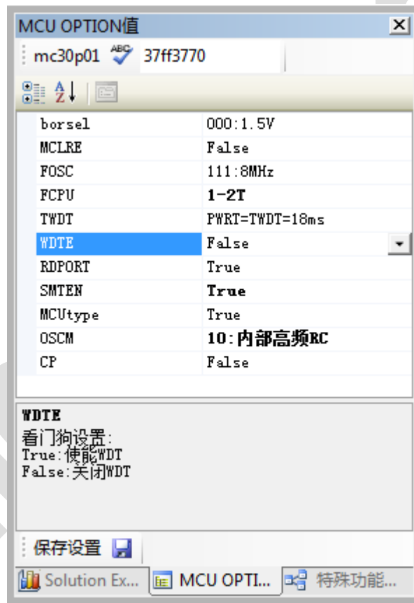
图 11 MCU OPTION 值设置
