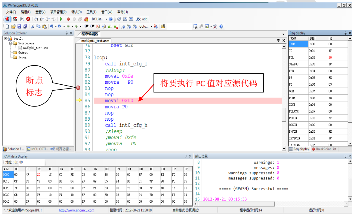
图 17 仿真模式下视图
