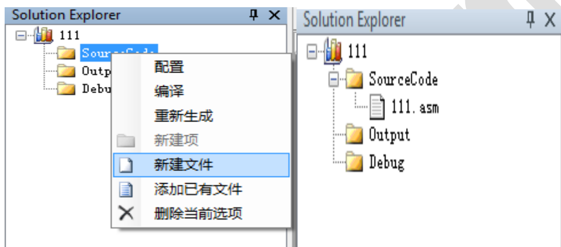
图 9 新建文件
