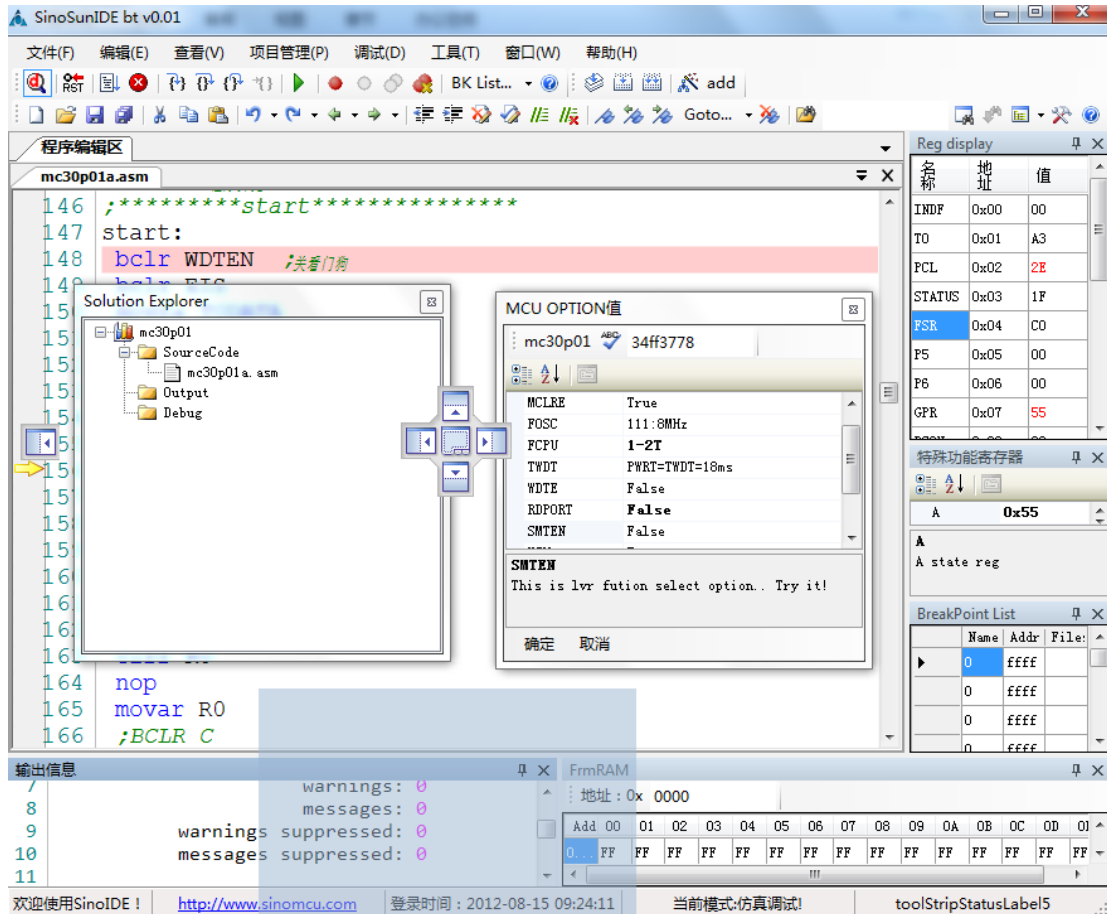
图 3 SinemcuIDE 主界面
