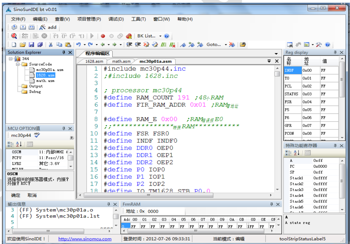
图 1 SinemcuIDE 界面
