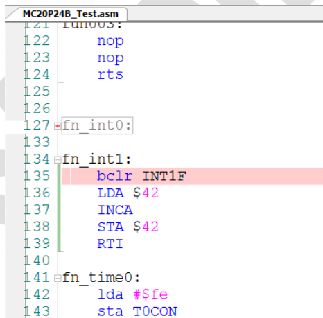
图 23 代码折叠
