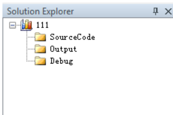
图 8 项目窗口
