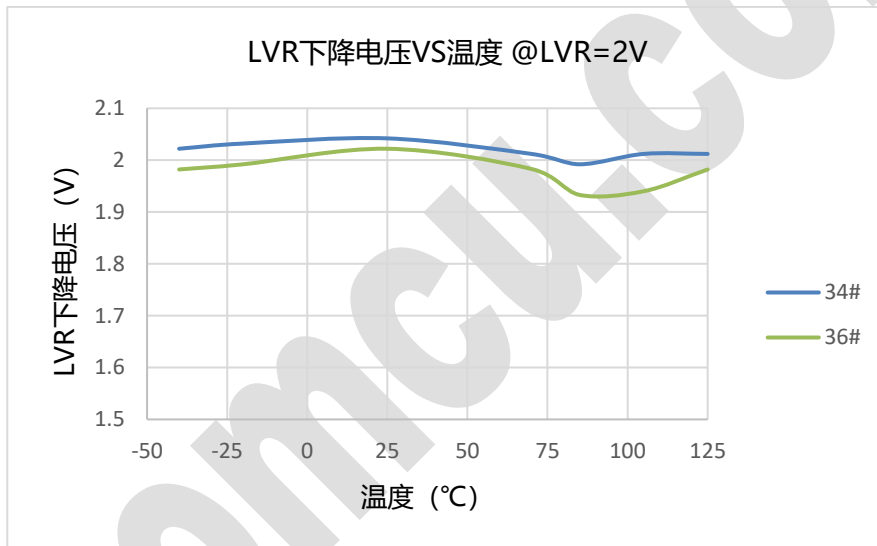
LVR 阈值电压 VS 温度
